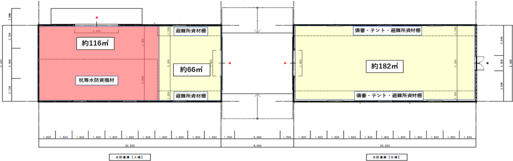
水防倉庫平面図 S=1:100 [北側 上向き 100mm = 1m]
