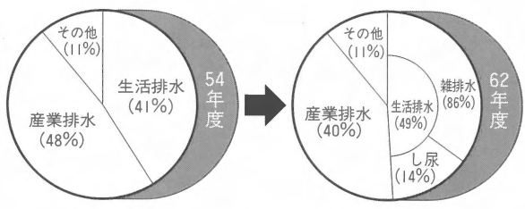
公共用水域に占める生活雑排水の汚濁割合 (COD)
